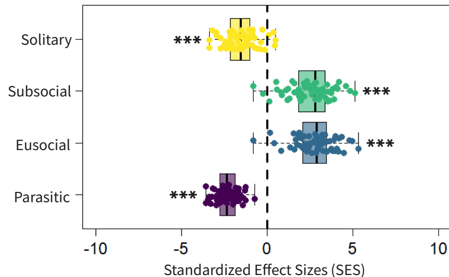
(d) Sociality
